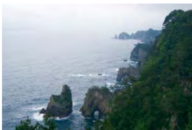
▲陸中海岸以峭壁及奇岩怪石為著稱。
